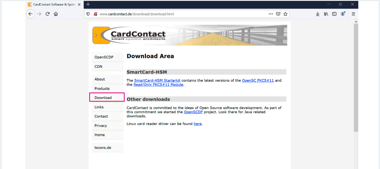
Abbildung 68: Downloadbereich
