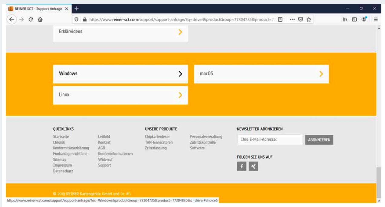
Abbildung 59: Betriebssystem auswählen
