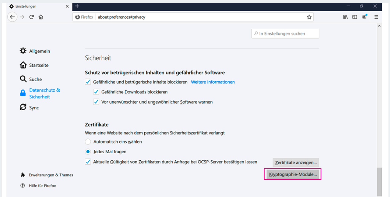
Abbildung 73: Browser-Einstellungen „Kryptographie-Module“
