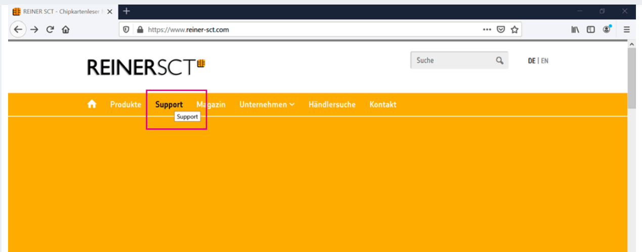
Abbildung 55: „Support“ auswählen
