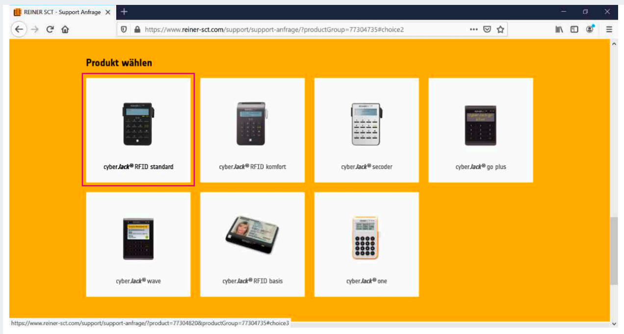
Abbildung 57: Produkt wählen
