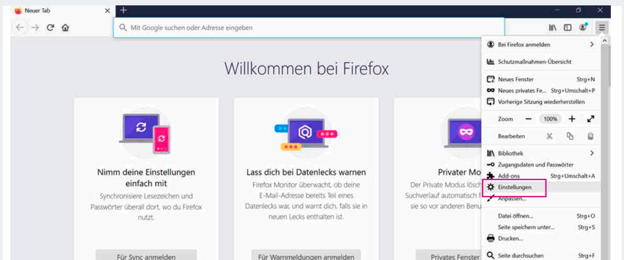
Abbildung 71: Browser-Einstellungen öffnen
