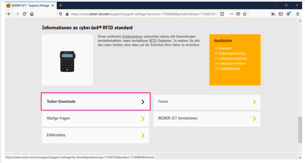
Abbildung 58: Treiber-Downloads
