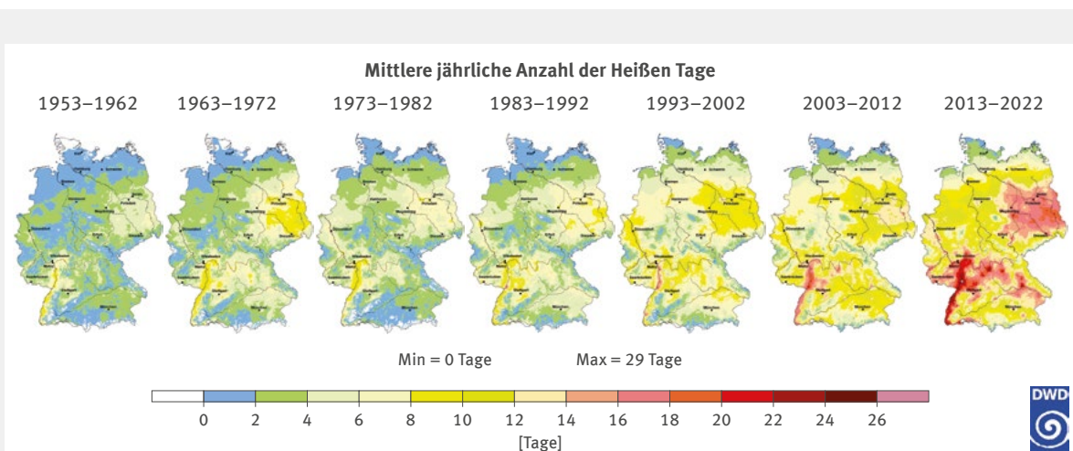
Abbildung 6: Mittlere jährliche Anzahl der Heißen Tage (Daten: DWD)
